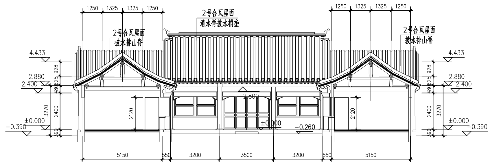
1-1剖面图 1: 100
