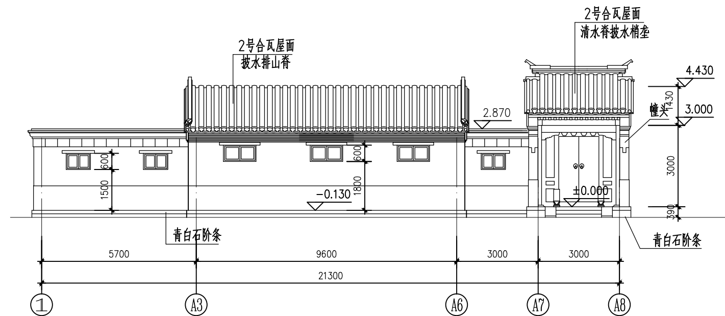
①—A8 立面图 1: 100
