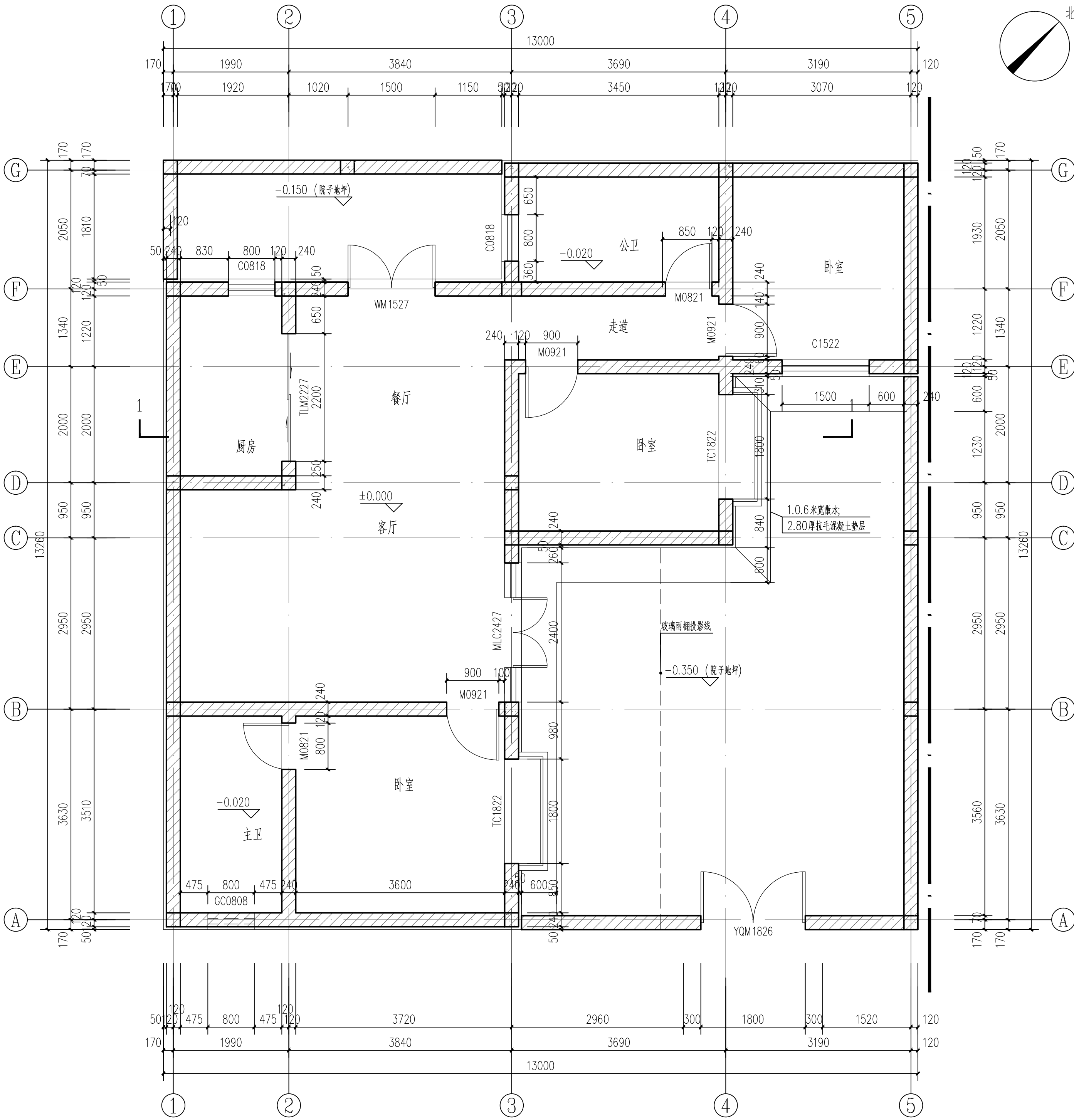
首层平面图 1:50
