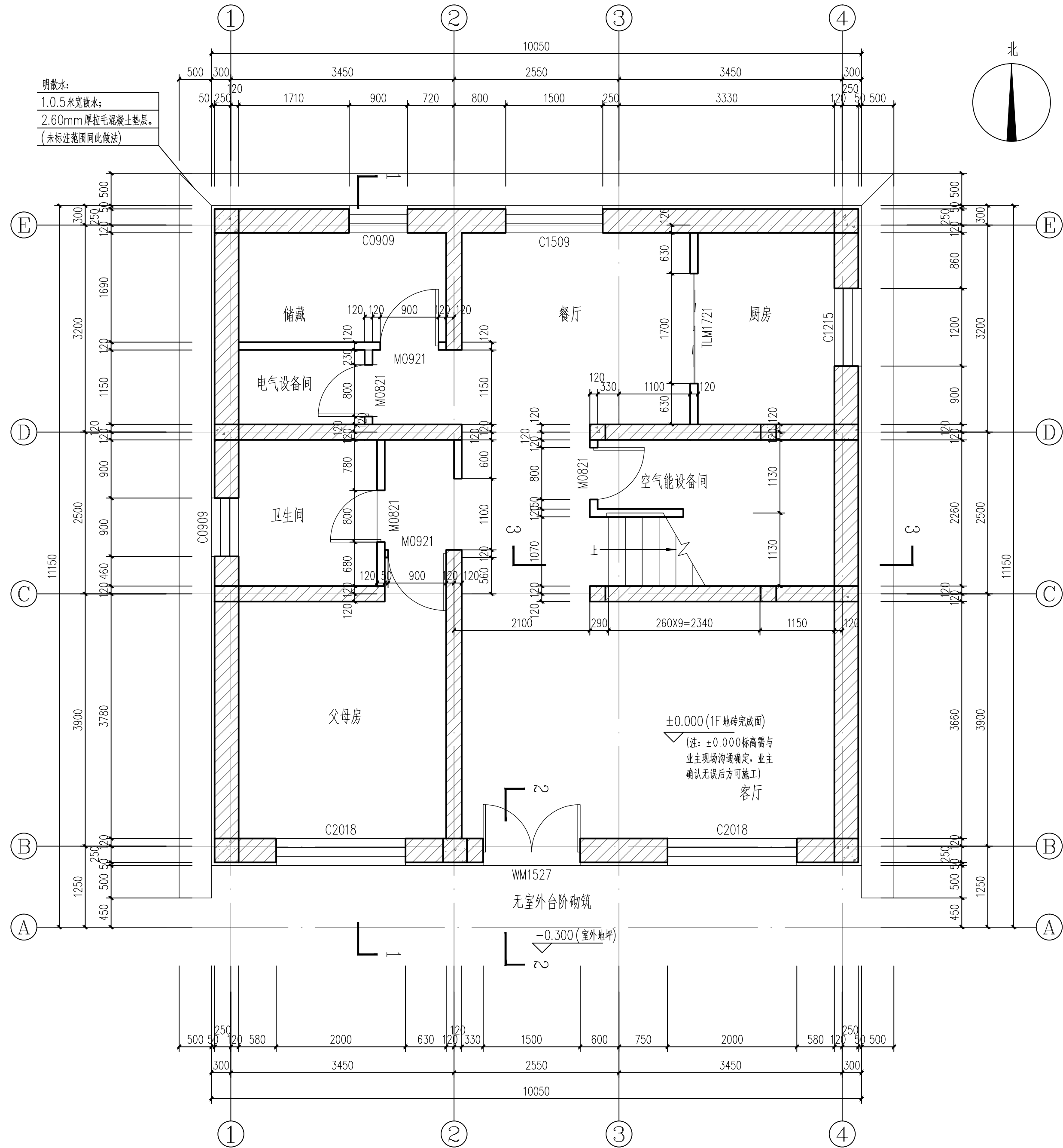
首层平面图 1:50
