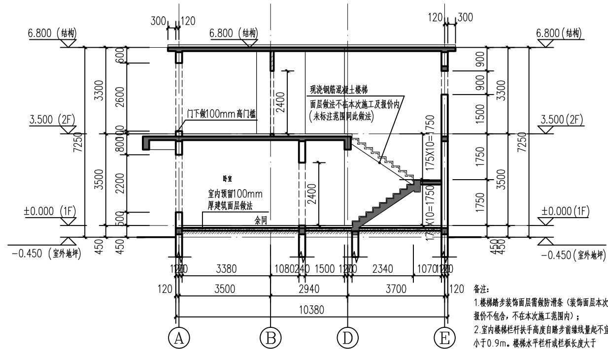
1-1 剖面图 1:100
