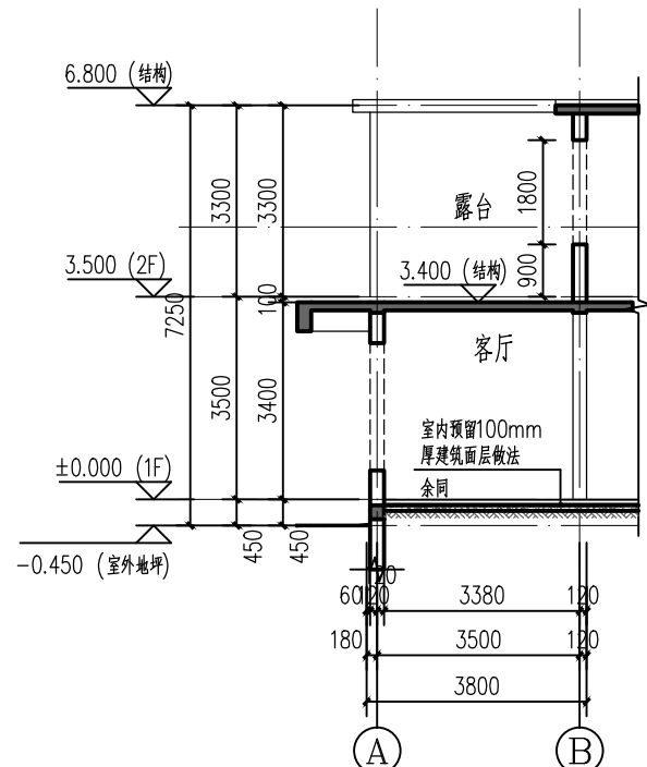
2-2 剖面图 1:100
