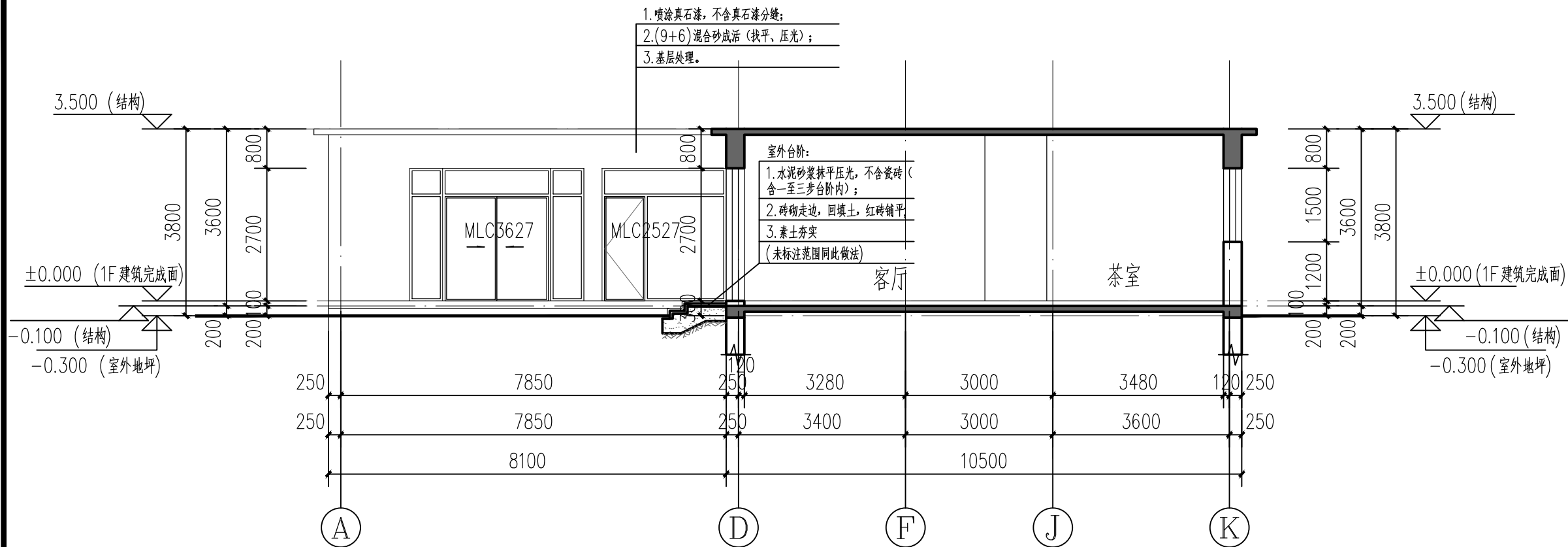
1-1 剖立面图 1:100
