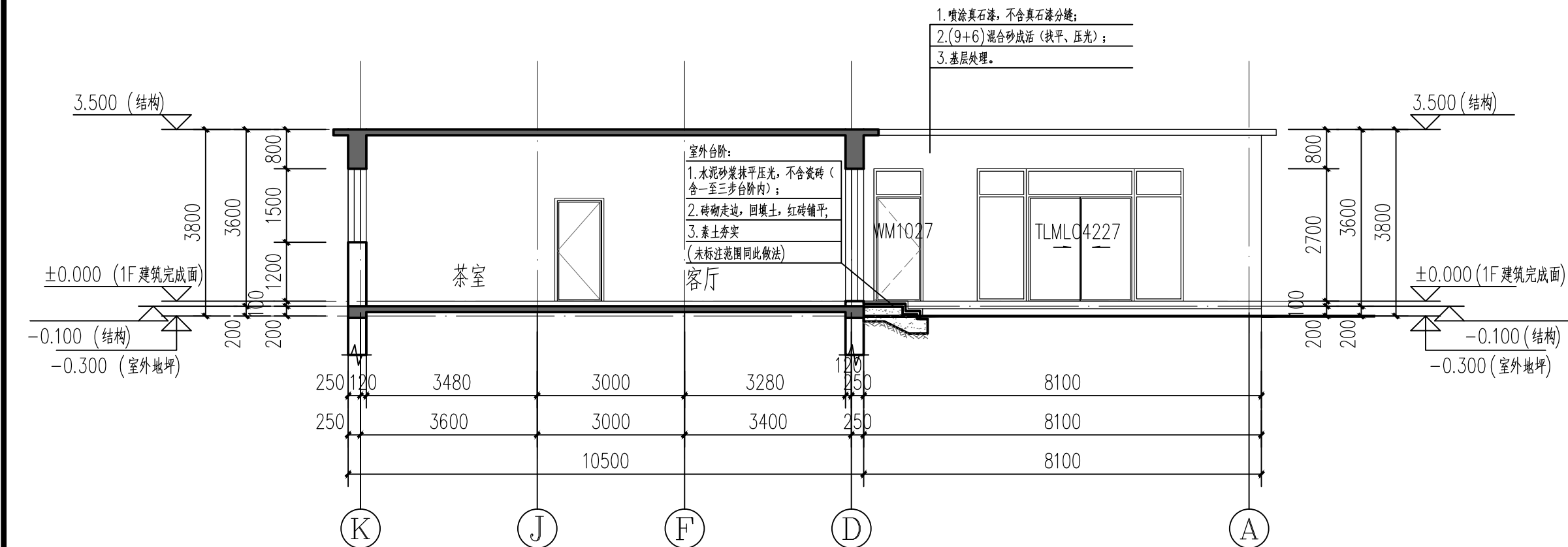
2-2 剖立面图 1:100
